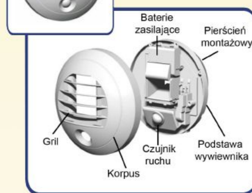
Wywiewnik stabilnego przepływu STABILVENT PIR z czujnikiem ruchu
