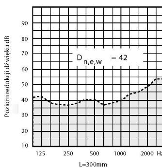
Tłumienie hałasu dla nawiewnika 100 Thermo dB (ref. 10 m 2 )
