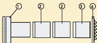
Tłumienie hałasu dla Fresh TL-80R dla L=400
