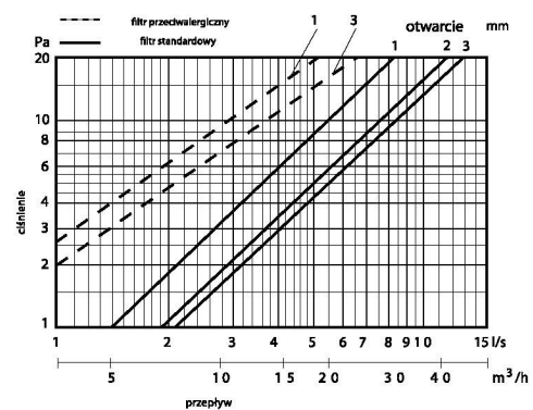
Wydajność TL80R
