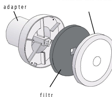
ochrona kondensacyjna
