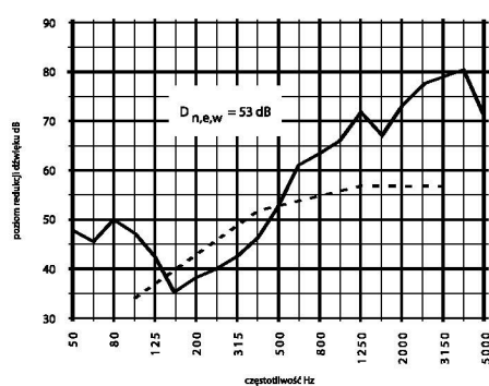
Tłumienie hałasu dla Fresh TL-80R dla L=400
