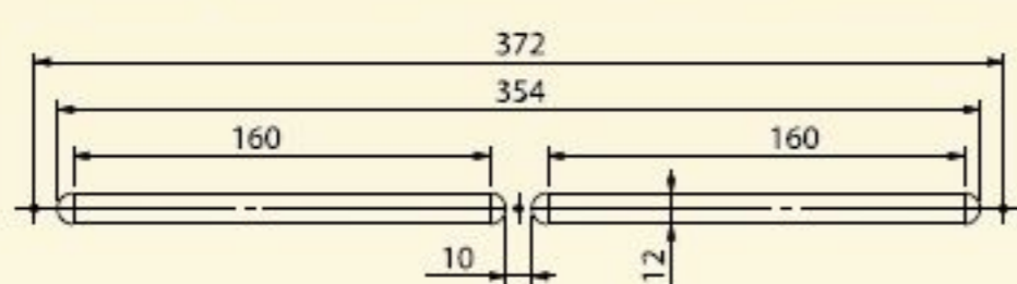
Wymiary otworów przelotowych i mocujących (mm)
